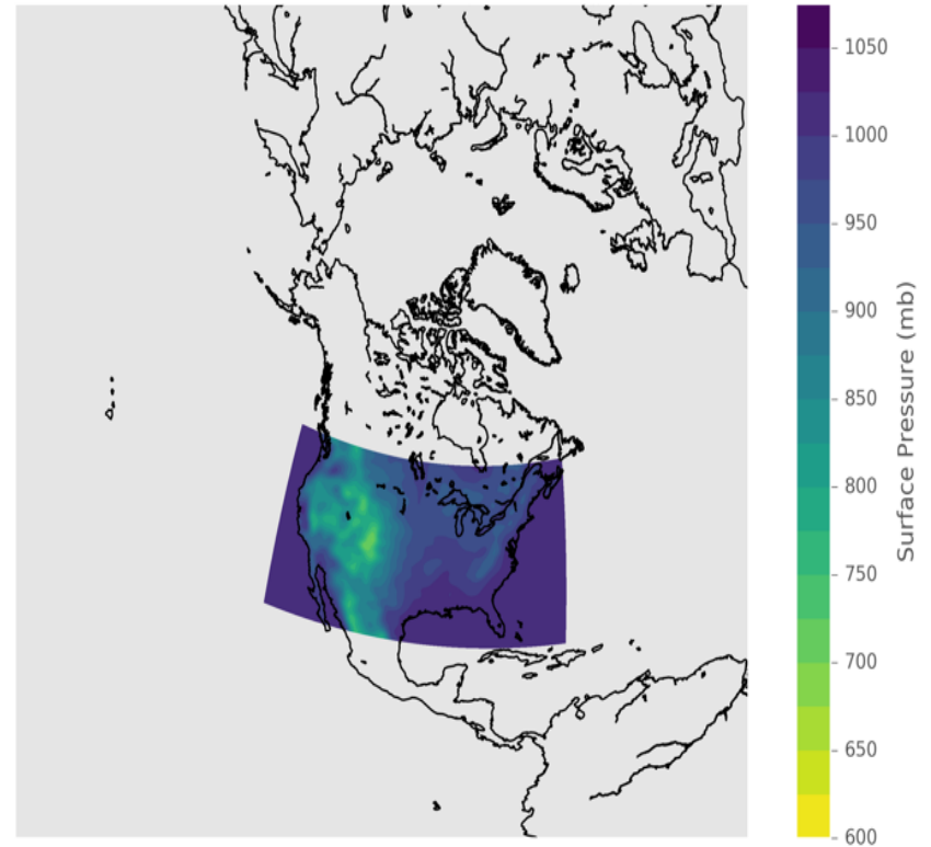
CMAQ
