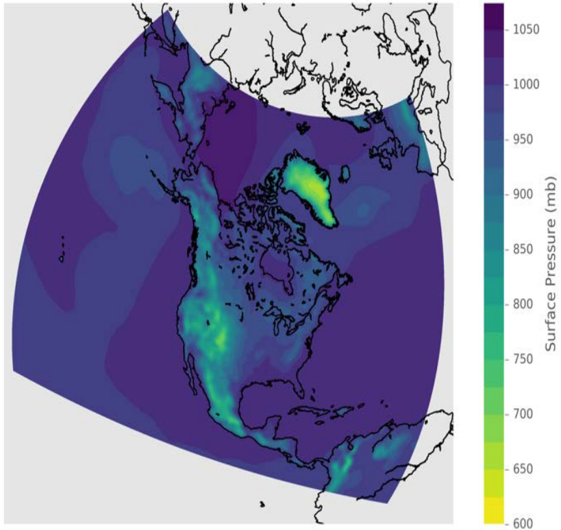
NMMB
